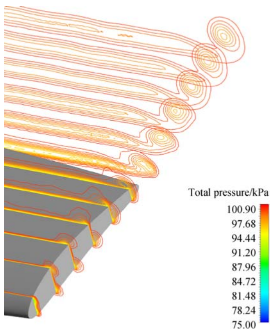
图 13 叶尖处截面总压等值线(Case 0)
