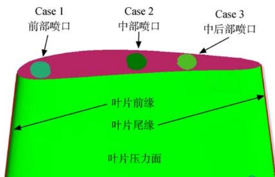
图 2 叶尖喷口位置
