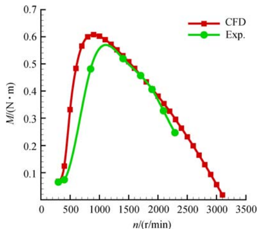
图6 风力机扭矩CFD计算结果与实验值比较
