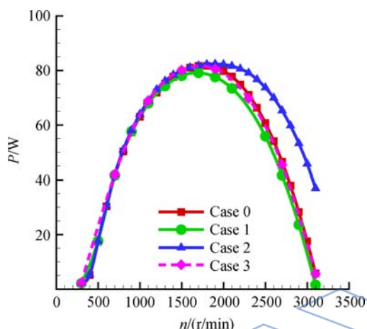
图 8 风力机功率随转速变化曲线
