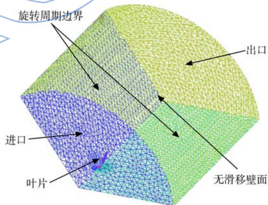
图 3 计算网格及边界设置图
