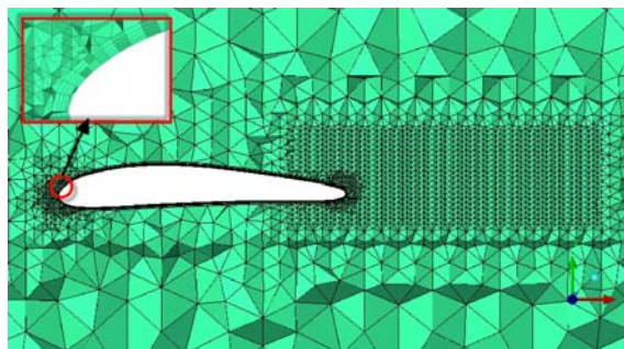
图 4 96% 叶高截面网格细节
