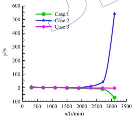
图 9 功率增长率随转速变化曲线
