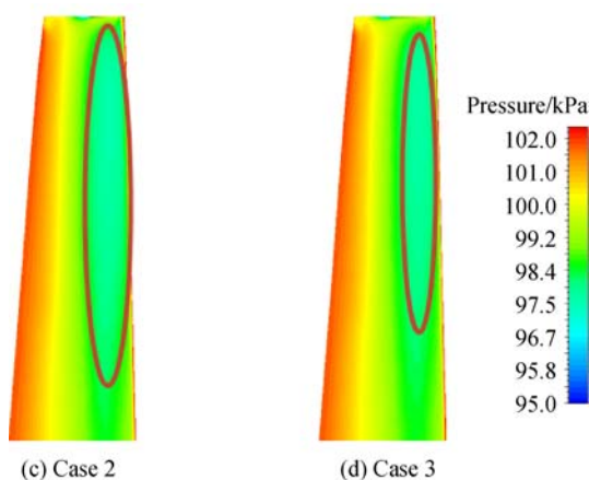
图 12 叶尖吸力面压力分布
