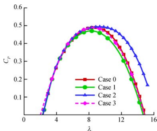
图 10 C_p - \lambda 曲线
