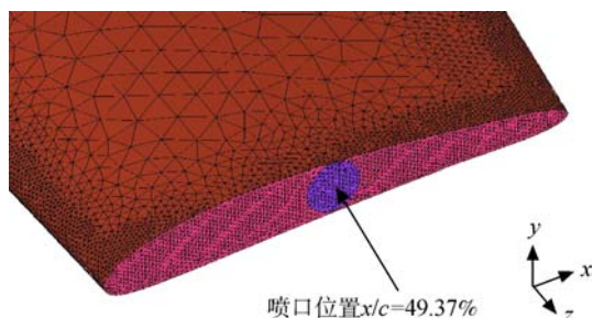
图5 叶尖表面网格分布(Case 2)
