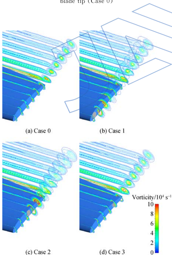
图 14 叶尖区域涡量等值线分布(Case 0~Case 3)
